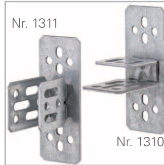
C-Profile Anschlüsse Nr. 1310 horizontal Nr. 1311 vertikal
